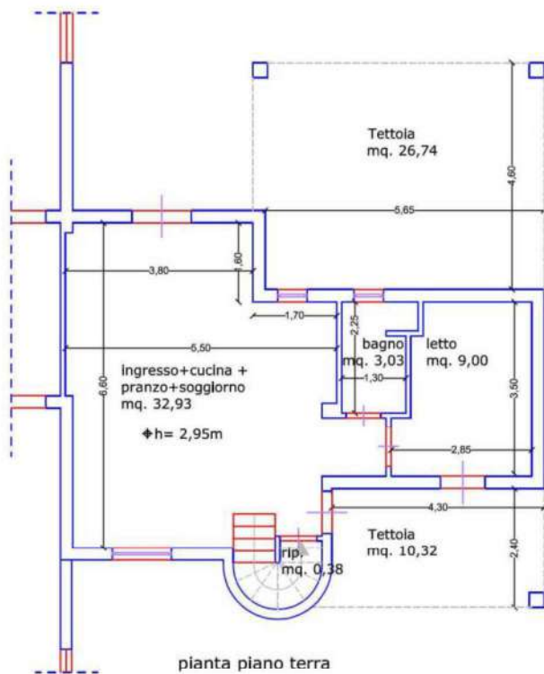
Immagine 2 (elaborato grafico del rilievo effettuato in data 06/02/2018)
