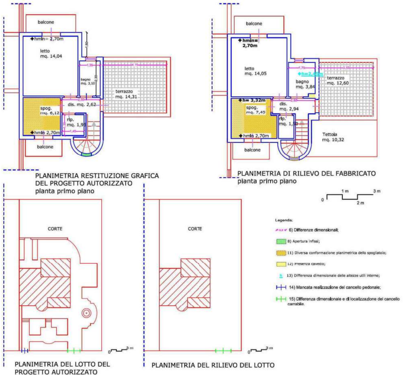
Immagine 24 (Raffronto piante primo piano tra lo stato dei luoghi alla data del sopralluogo e la restituzione grafica del progetto autorizzato e raffronto planimetrie del lotto tra lo stato dei luoghi alla data del sopralluogo e la planimetria del lotto del progetto autorizzato)
