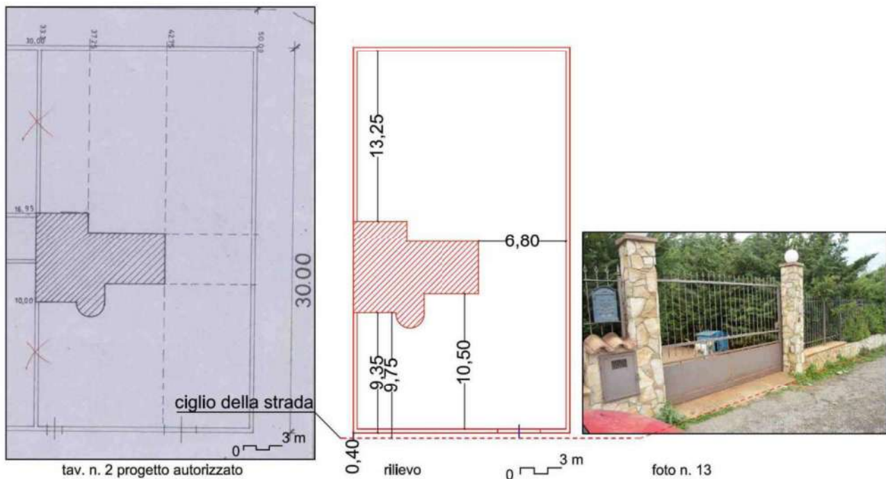
Immagine 25 (distanze del fabbricato dai confini e dal ciglio stradale)
