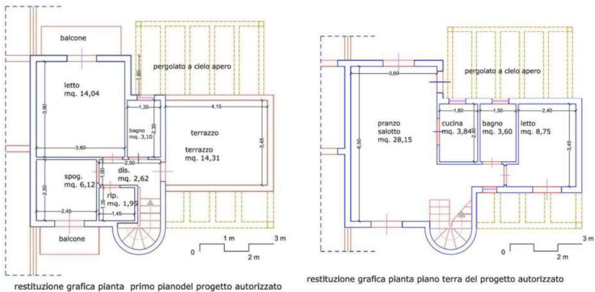
Immagine 13 (restituzione grafica del progetto autorizzato)
