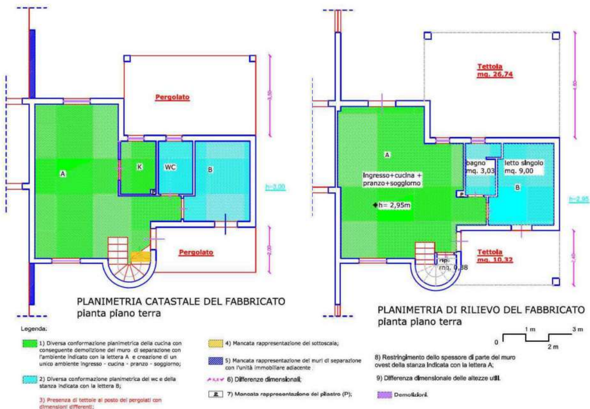
Immagine 8 (Raffronto delle piante del piano terra tra lo stato dei luoghi alla data del sopralluogo e la planimetria catastale)
