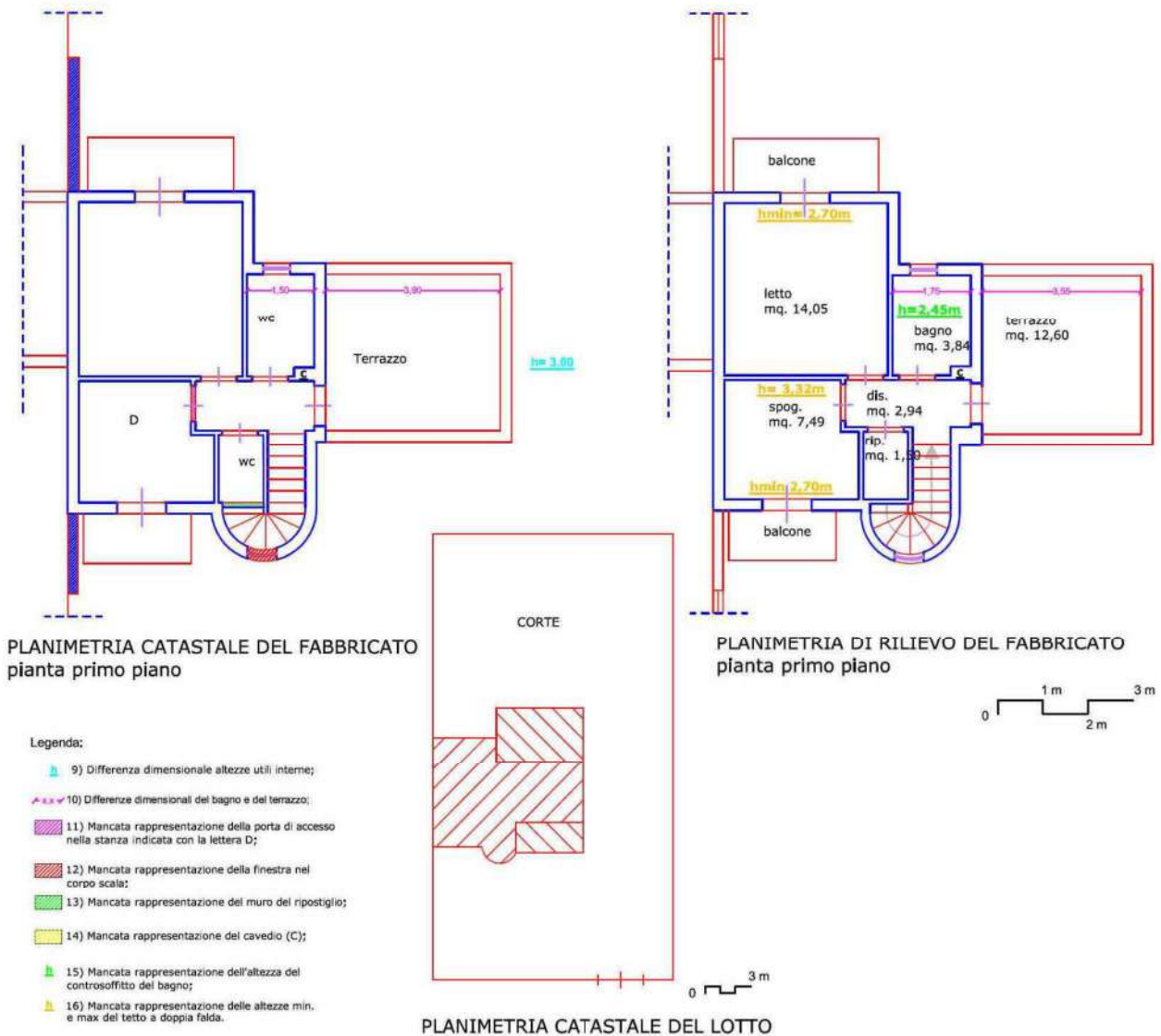
Immagine 9 (Raffronto delle piante primo piano tra lo stato dei luoghi alla data del sopralluogo e la planimetria catastale)
