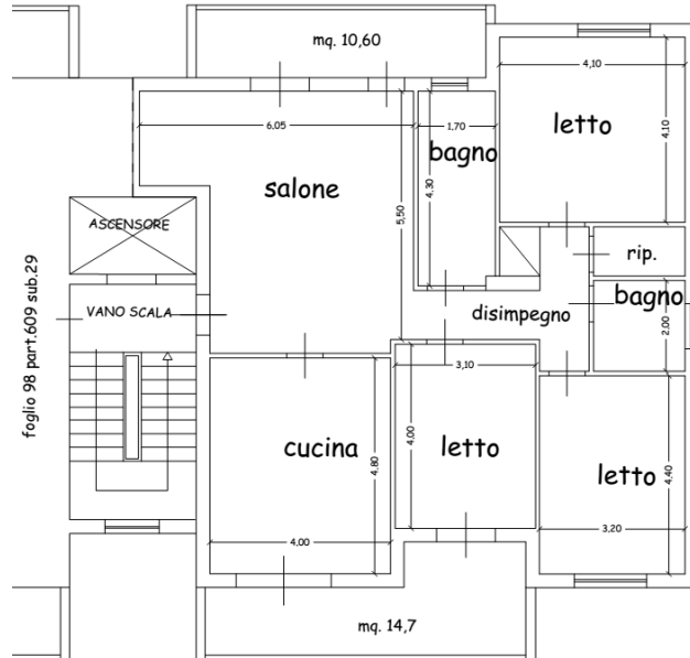
PIANTA PIANO PRIMO PAL. B foglio 98 part.609 sub.28
