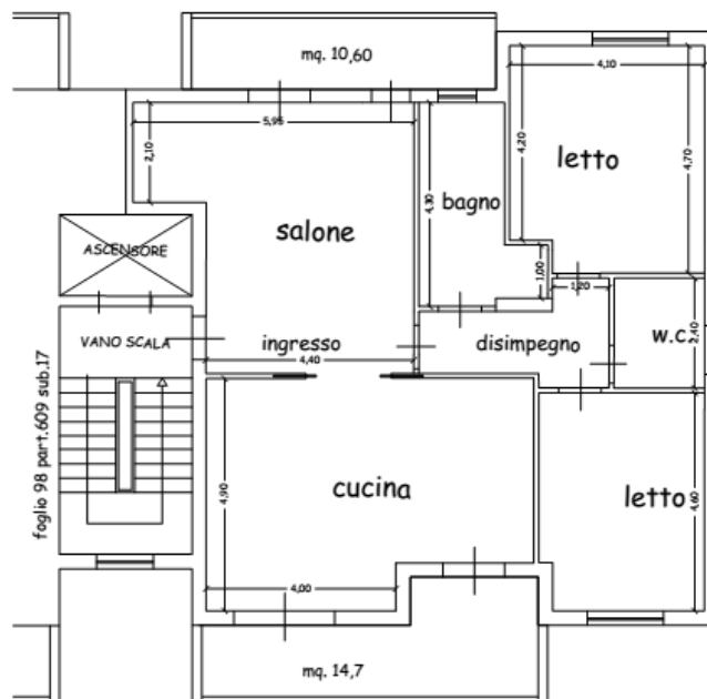
PIANTA PIANO TERZO PAL. A. foglio 98 part.609 sub.16
