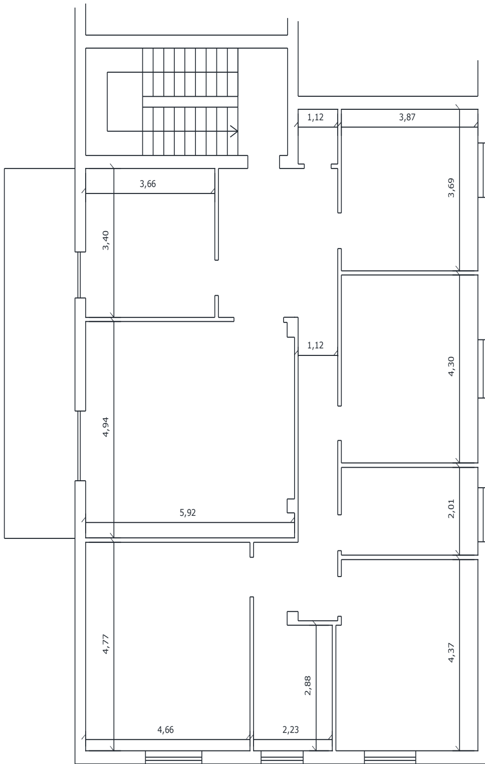
Planimetria piano primo Unità immobiliare Sub 9/11
