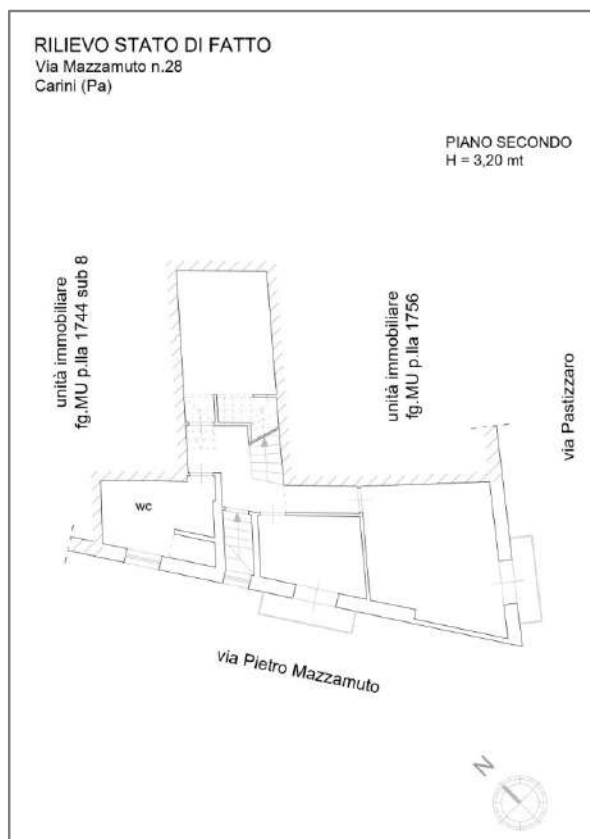
Rilievo dello stato di fatto del piano secondo
