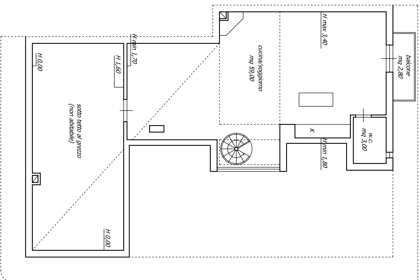
PIANO SECONDO H = media 2,60
