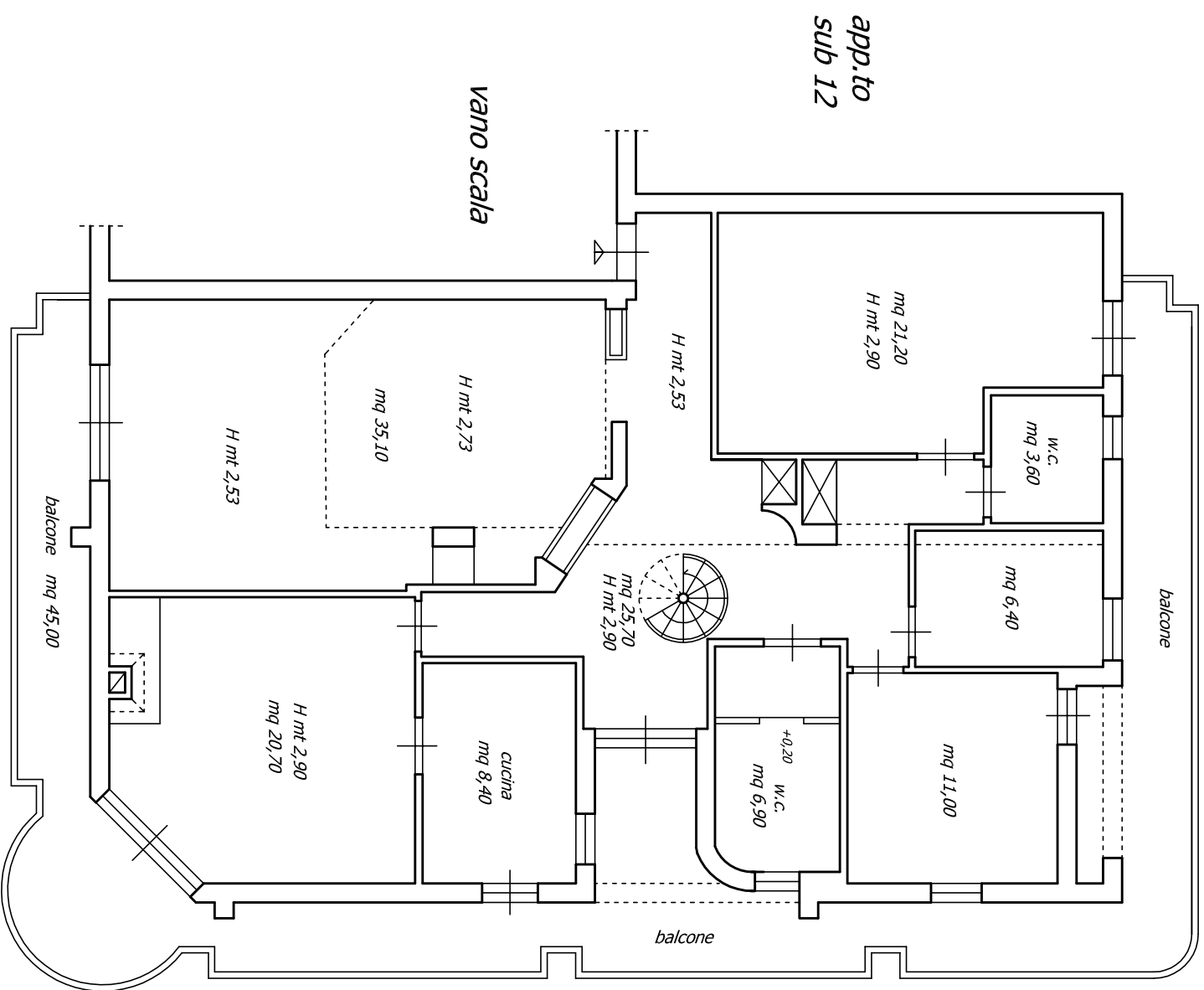
PIANO PRIMO H = mt 2,90
