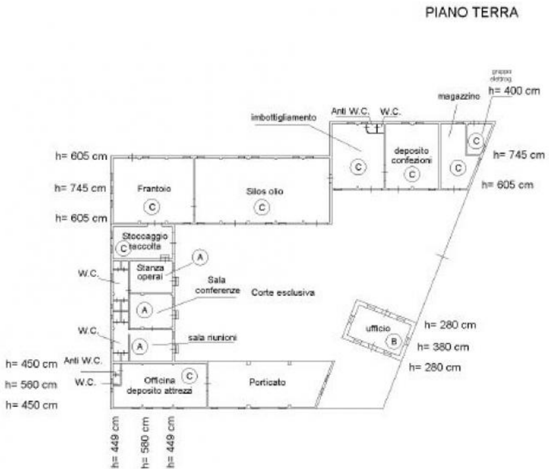
Centro Aziendale - Pianta del centro aziendale per la trasformazione ed imbottigliamento delle olive.
