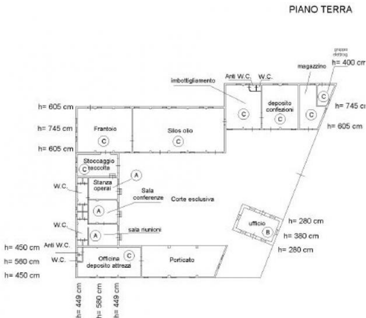
Pianta generale del Centro Aziendale.
