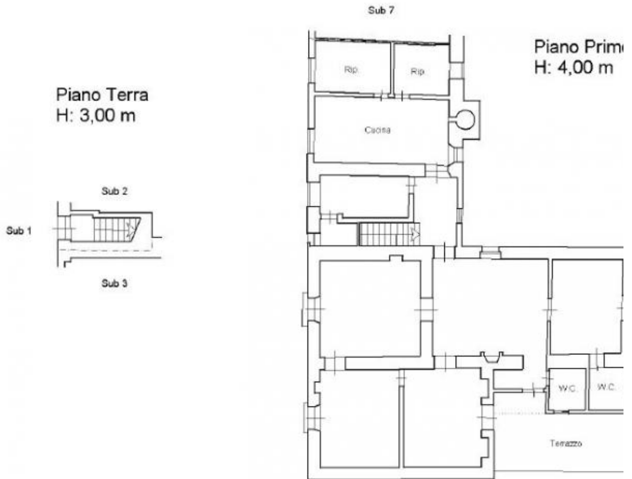
Pianta primo piano, sub 6, edificio "B".
