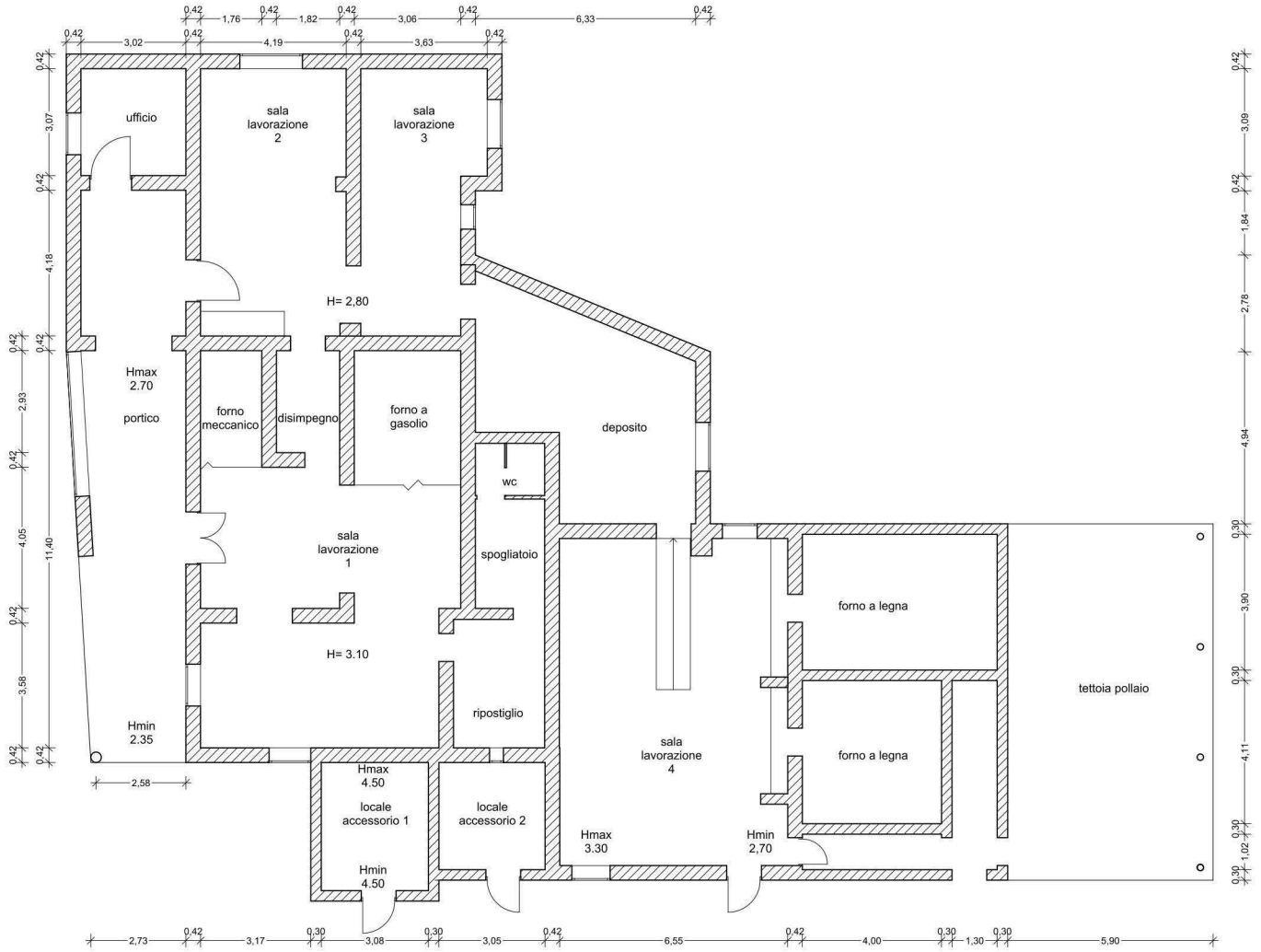
PLANIMETRIA STATOATTUALE PIANO TERRA scala 1:100
